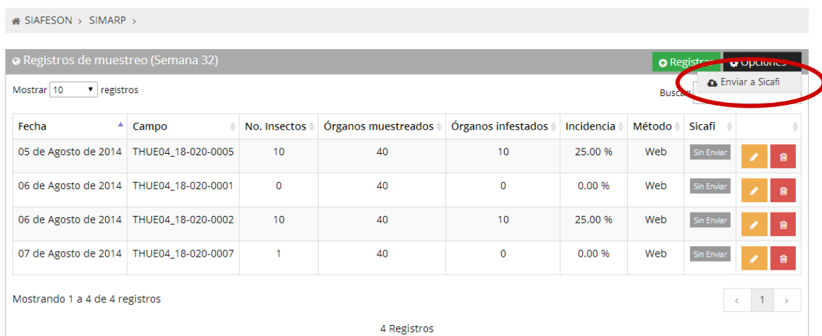
Fig. 22. Ubicación en la tabla del botón para “Enviar a SICAFI” información registrada.
